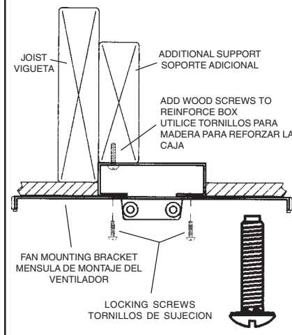
SECURING CEILING BOX BETWEEN JOISTS COMO ASEGURAR LA CAJA DE TECHO INSTALADA ENTRE VIGUETAS
